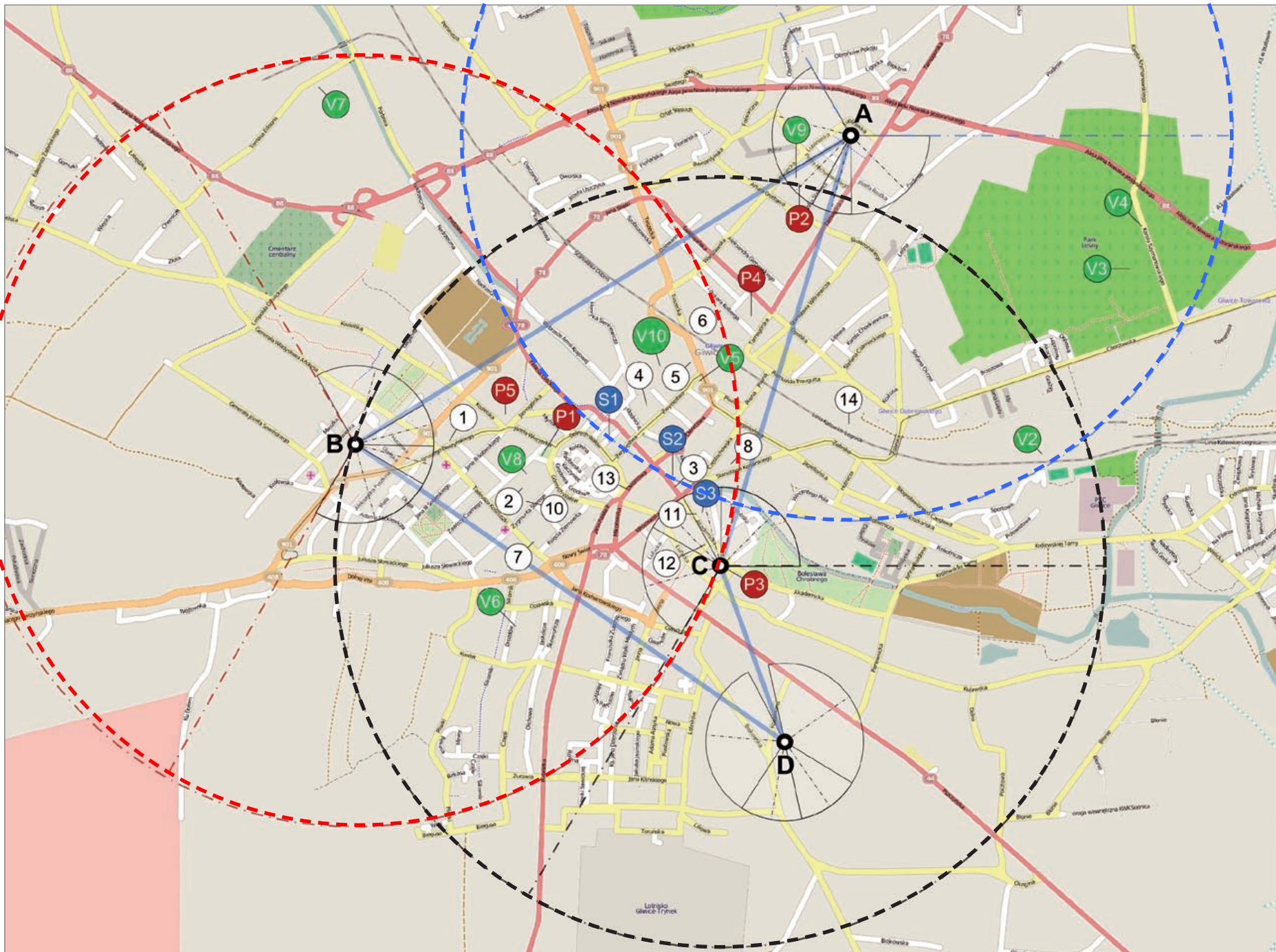
Rozmieszczenie i zasięg oddziaływania stacji bazowych umożliwiających emisję sygnału radiowego. Okręgi wyznaczają teren, na którym możliwe jest uruchomienie monitoringu, HotSpotów oraz innych usług.
