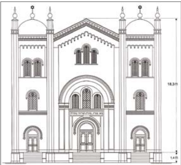
Dawna synagoga przy placu Inwalidów Wojennych, opracowanie – dr inż. Zbigniew Jura, na podstawie pomiarów fundamentów i fotogrametrii
